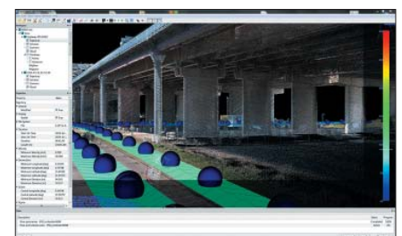
Комбинация из 32 лазеров дает оптимальное покрытие объекта
