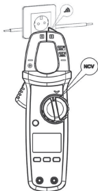
Рис. 5 Бесконтактное обнаружение переменного напряжения
