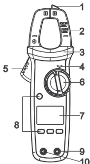
Рис.1 Общее устройство
