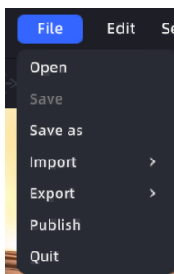
Меню «Файл»
