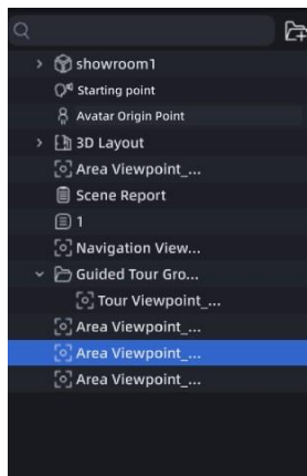
Список ассетов
