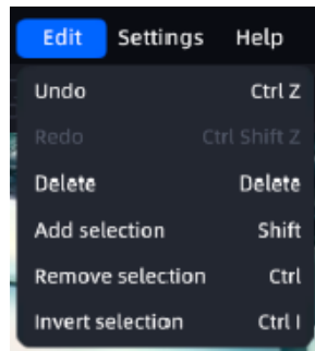
Меню «Правка»
