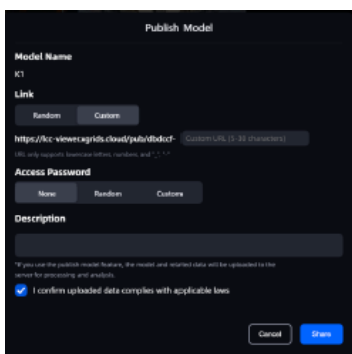
Диалог публикации
