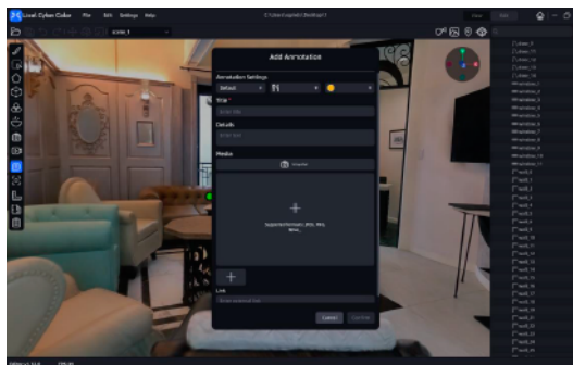
Добавление аннотации
