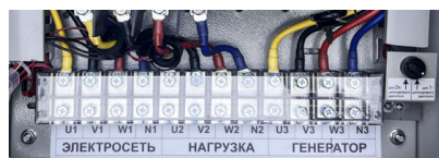
ДОПУСТИМЫЕ КЛЕММЫ ДЛЯ ПОДКЛЮЧЕНИЯ ТРЕХФАЗНОГО БЛОКА АВТОЗАПУСКА
